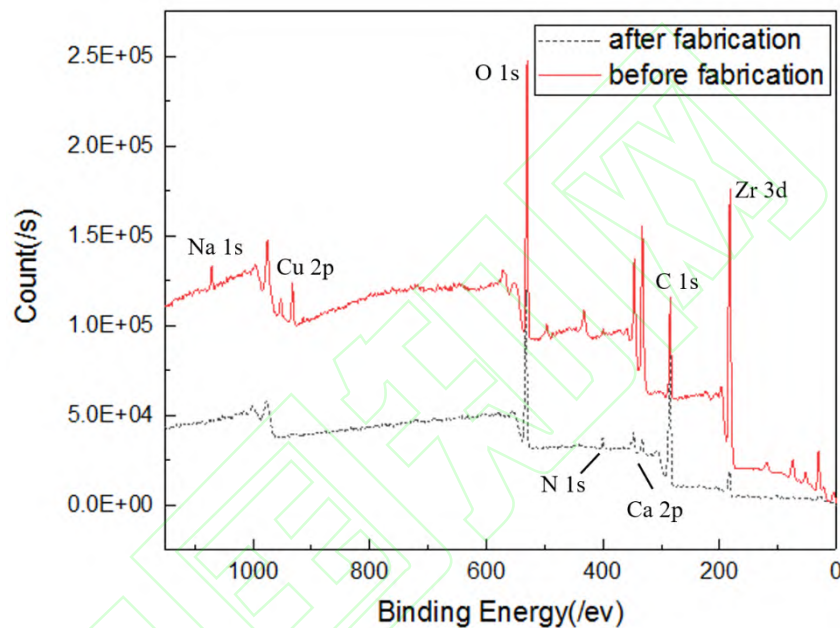
图 3 未加工表面和加工后直线结构表面 XPS 全谱图
