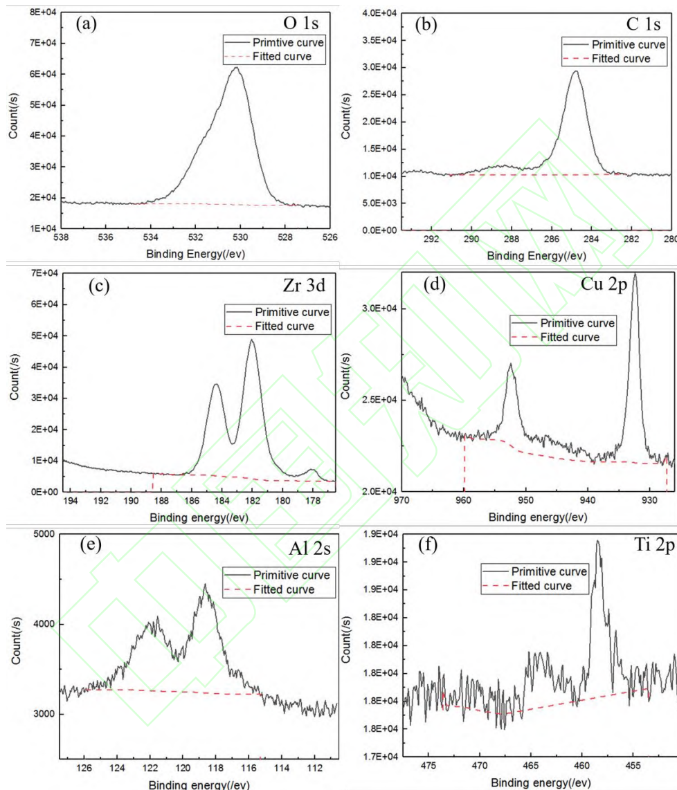
图 4 未加工抛光表面不同元素的 XPS 谱图及分峰示意图
