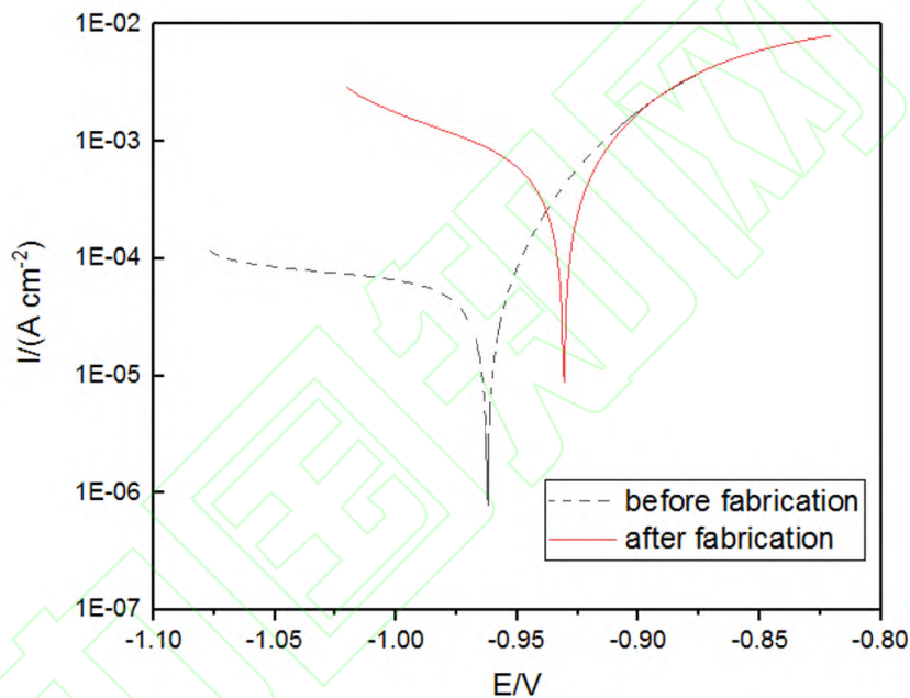
图 6 加工前后动电位极化曲线图
